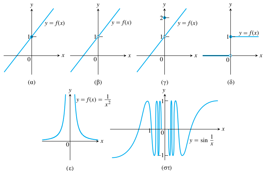
ΣΧΗΜΑ 1.50 Η συνάρτηση (α) είναι συνεχής στο x = 0 , κάτι που δεν ισχύει για τις συναρτήσεις (β) έως (στ).
