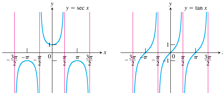
ΣΧΗΜΑ 1.34 Γραφικές παραστάσεις των συναρτήσεων \sec x και \tan x . (Παράδειγμα 8)
