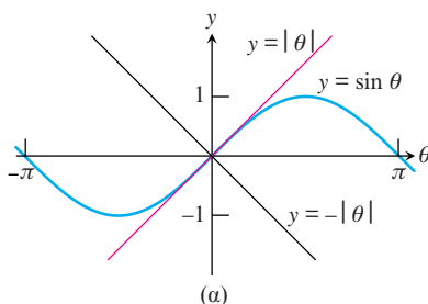
ΣΧΗΜΑ 1.19 Το θεώρημα «σάντουιτς» επαληθεύει ότι
