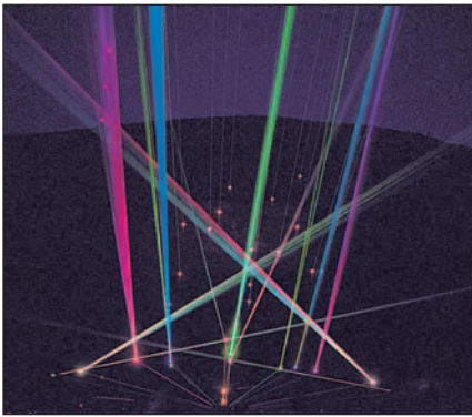
ΣΧΗΜΑ 1.44 Μια από τις συνέπειες της κατανόησης της φύσεως του ατόμου ήταν και η εφεύρεση του λείζερ.
