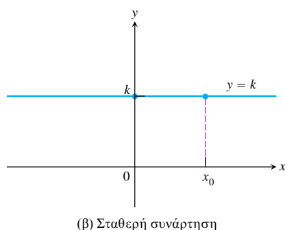
ΣΧΗΜΑ 1.7 Οι συναρτήσεις του Παραδείγματος 6.
