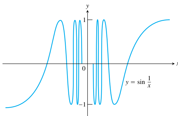
ΣΧΗΜΑ 1.23 Η συνάρτηση y = \sin(1/x) δεν έχει ούτε δεξιό ούτε αριστερό όριο καθώς το x τείνει στο μηδέν. (Παράδειγμα 9)
