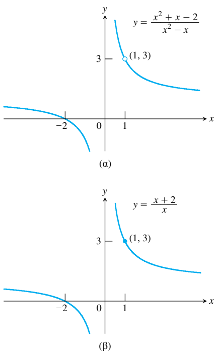
ΣΧΗΜΑ 1.15 Η γραφική παράσταση της f(x) = (x^2 + x - 2)/(x^2 - x) στο (α) συμπίπτει με αυτήν της g(x) = (x + 2)/x στο (β), με εξαίρεση το σημείο x = 1 , όπου η f δεν ορίζεται. Οι δύο συναρτήσεις έχουν κοινό όριο καθώς x \rightarrow 1 .
