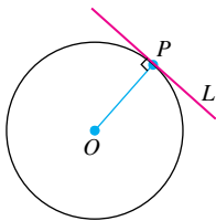
ΣΧΗΜΑ 1.58 Η ευθεία L εφάπτεται του κύκλου στο σημείο P αν διέρχεται από το P κάθετα στην ακτίνα OP .
