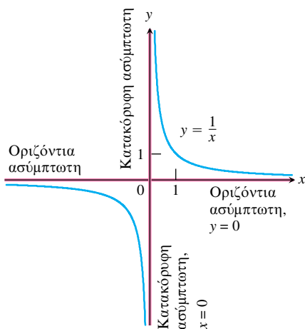
ΣΧΗΜΑ 1.30 Οι άξονες συντεταγμένων αποτελούν τις ασύμπτωτες των κλάδων της υπερβολής y = 1/x .
