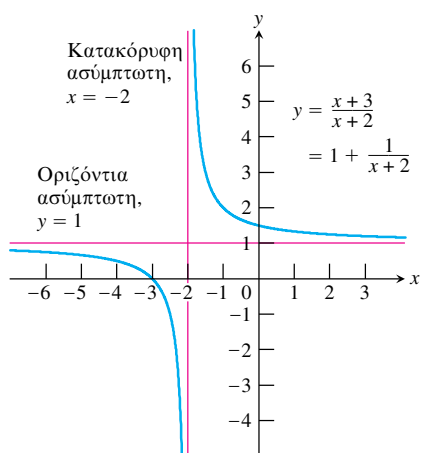
ΣΧΗΜΑ 1.32 Οι ευθείες y = 1 και x = -2 είναι ασύμπτωτες της καμπύλης y = (x + 3)/(x + 2) . (Παράδειγμα 6)
